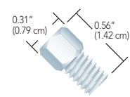
C-235 1/4-28 Stainless Steel Nut for 1/8" OD tubing
